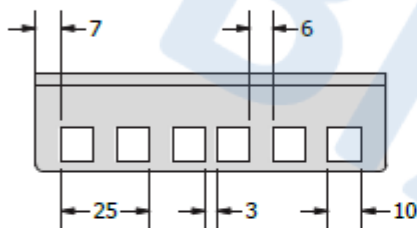
Vista dall'alto
